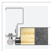
FB Stahltürrahmen
