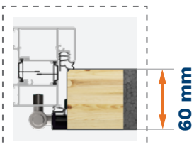
ALUTHERM 60* Türrahmen
