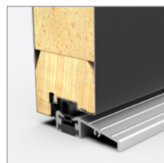
4 Fälze im Türblatt
