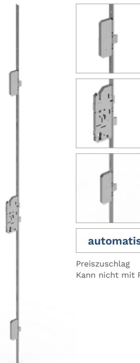
automatisches 3-Riegel-Schloss
