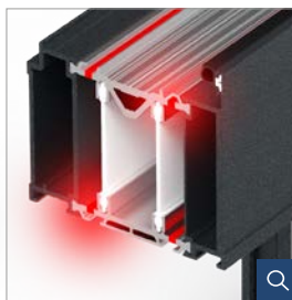
Kompensationsthermik
