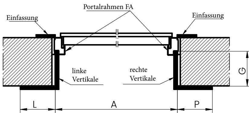
HORIZONATALSCHNITT
