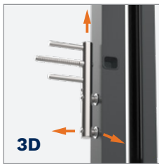
3D panty s krytkami v barvě kování
