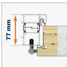
Zárubeň ALUTHERM 75
