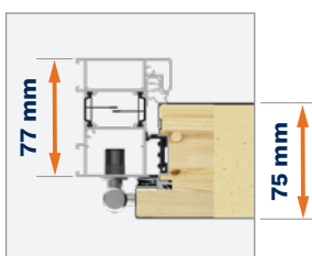
Zárubeň ALUTHERM 75
