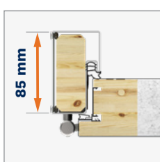
Zárubeň DUOTHERM 60
