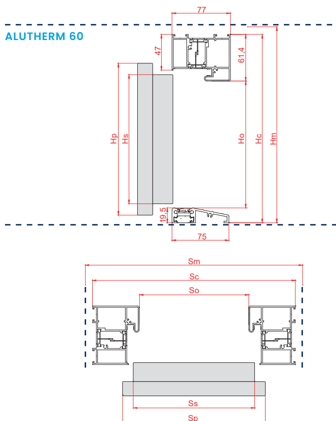
DUOTHERM 60
