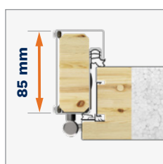
Zárubeň DUOTHERM 75
