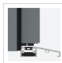
4 zárubně křídla
