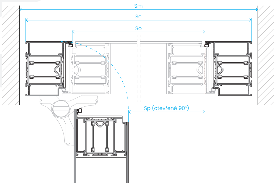
Horizontální řez
