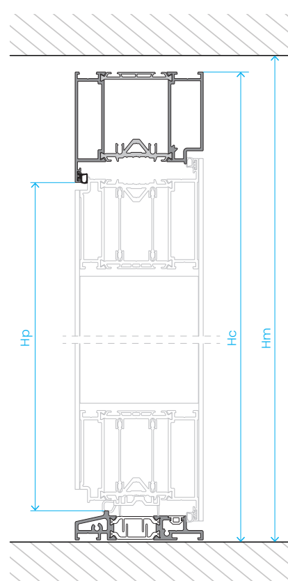
Vertikální řez
