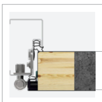
Дверна коробка PERFOTHERM 60
