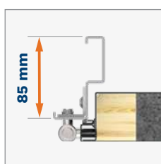
Ościeżnica stalowa FN
