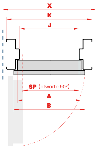
PRZĘKRÓJ POZIOMY
