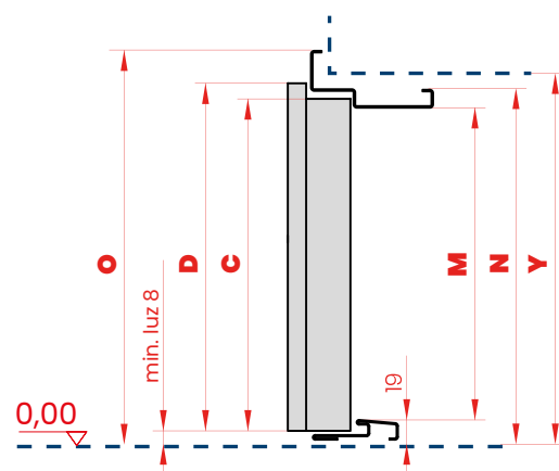
PRZEKRÓJ PIONOWY
