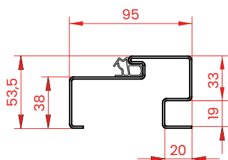
PROFIL OŚCIEŻNICY
