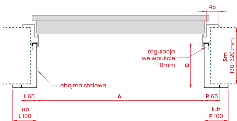
PRZEKRÓJ POZIOMY
