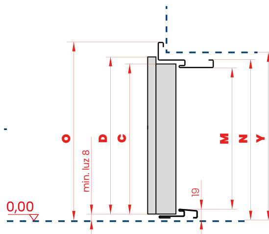
PRZEKRÓJ PIONOWY
