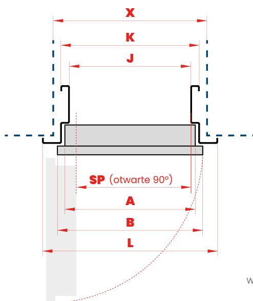
PRZEKRÓJ POZIOMY
