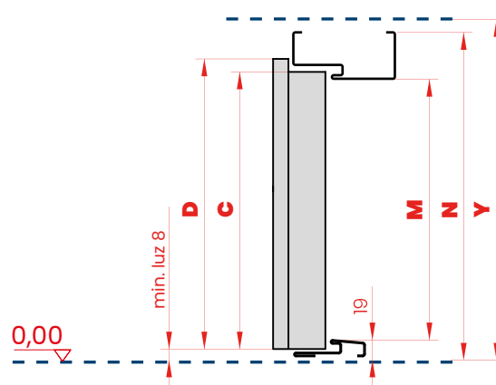
PRZEKRÓJ PIONOWY
