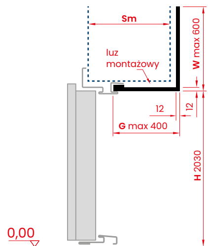
PRZEKRÓJ PIONOWY
