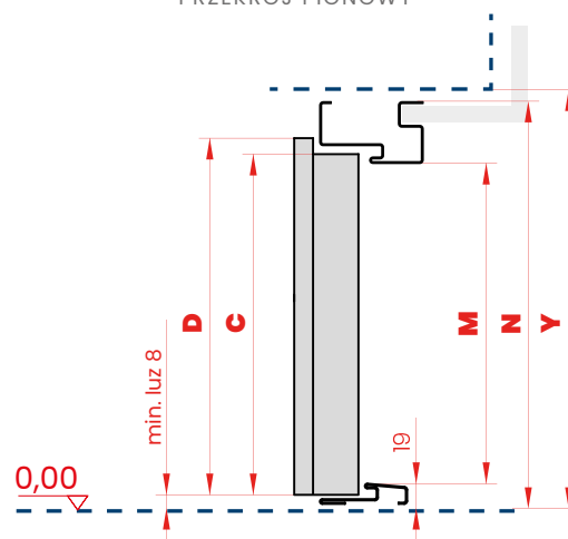
PRZEKRÓJ PIONOWY
