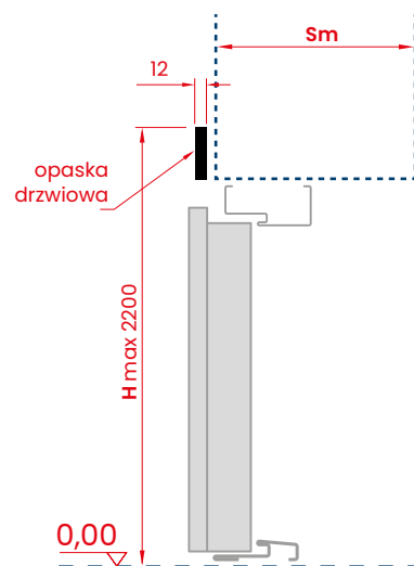
PRZEKRÓJ PIONOWY
