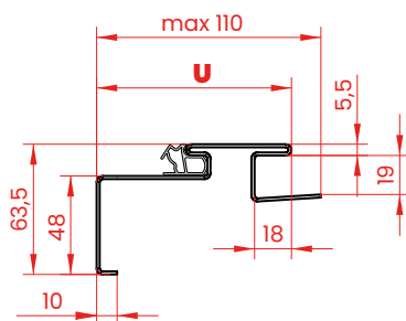
PROFIL OŚCIEŻNICY
