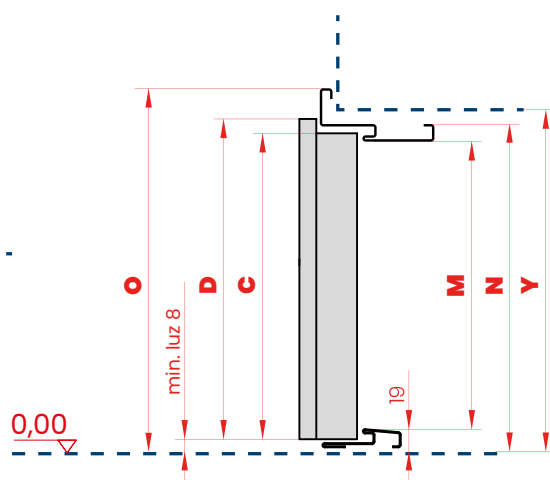
PRZEKRÓJ PIONOWY
