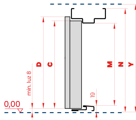
PRZEKRÓJ PIONOWY
