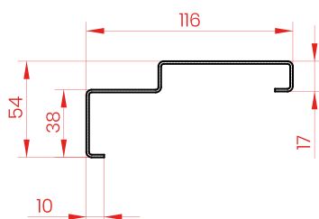
PROFIL OŚCIEŻNICY
