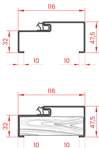
PROFIL OŚCIEŻNICY
