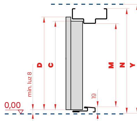
PRZĘKRÓJ PIONOWY
