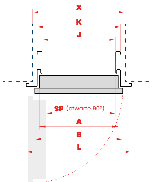
PRZEKRÓJ POZIOMY
