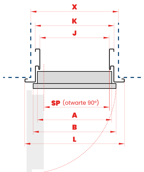
PRZEKRÓJ POZIOMY
