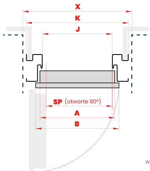
PRZEKRÓJ POZIOMY
