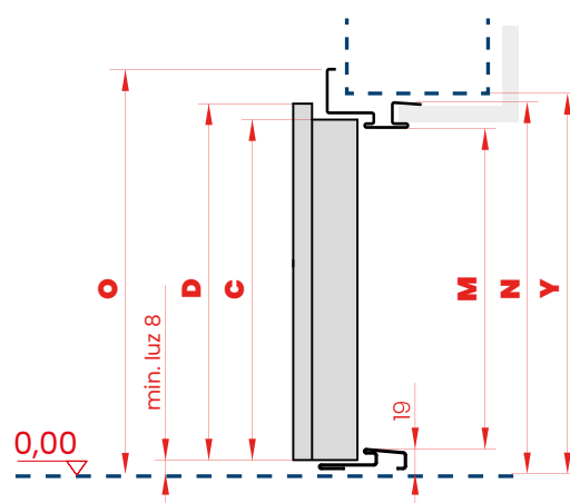
PRZEKRÓJ PIONOWY
