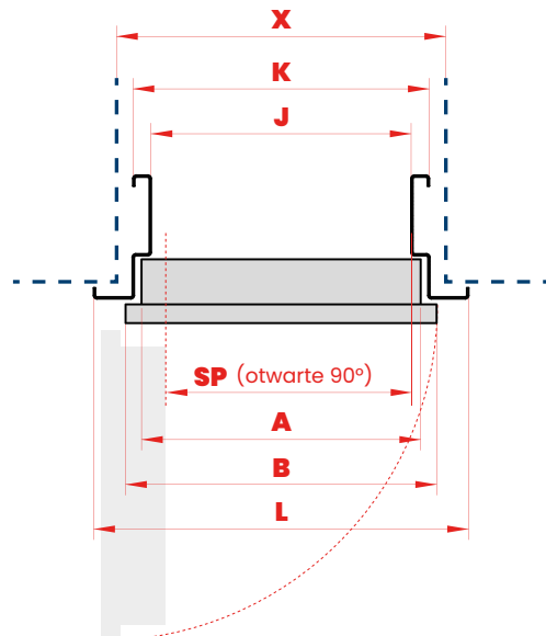
PRZEKRÓJ POZIOMY
