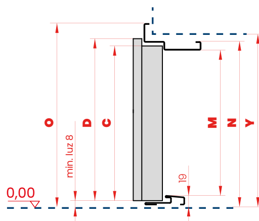
PRZEKRÓJ PIONOWY
