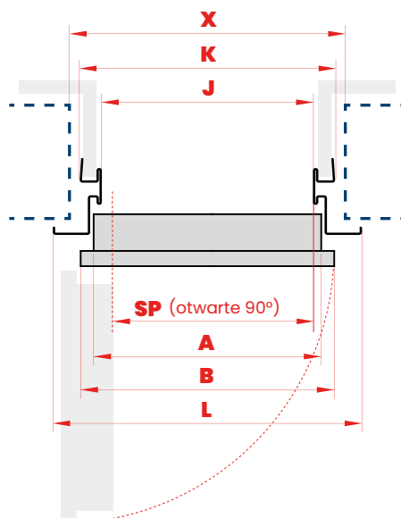
PRZEKRÓJ POZIOMY
