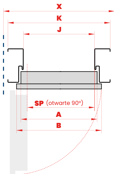
PRZEKRÓJ POZIOMY
