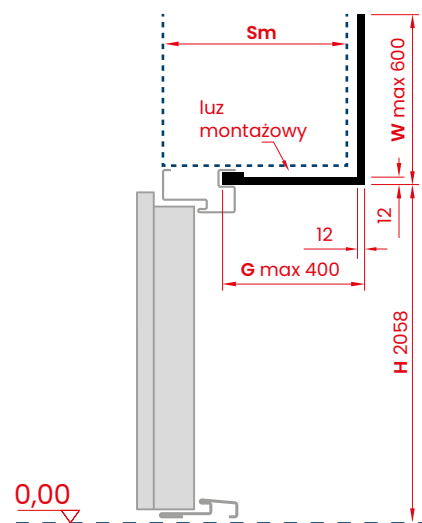
PRZEKRÓJ PIONOWY
