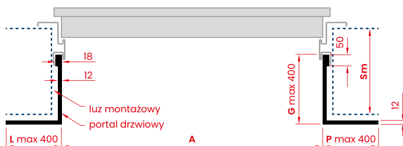
PRZEKRÓJ POZIOMY
