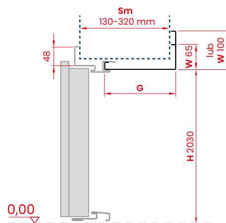
PRZEKRÓJ PIONOWY
