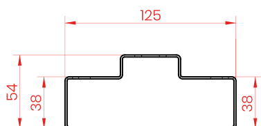
PROFIL OŚCIEŻNICY
