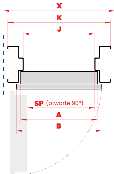
PRZEKRÓJ POZIOMY
