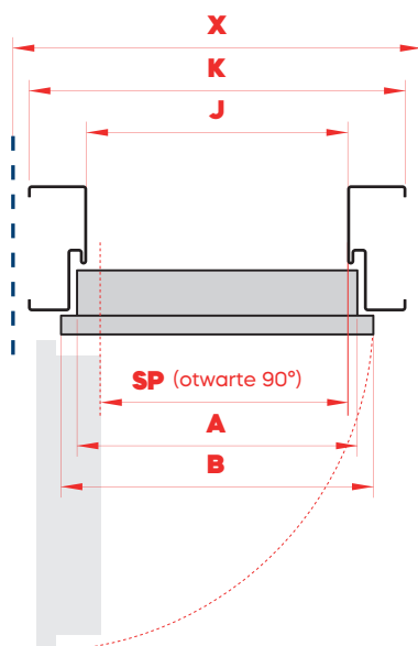
PRZEKRÓJ POZIOMY
