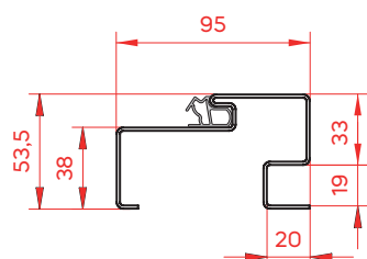
PROFIL OŚCIEŻNICY
