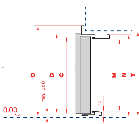
PRZEKRÓJ PIONOWY
