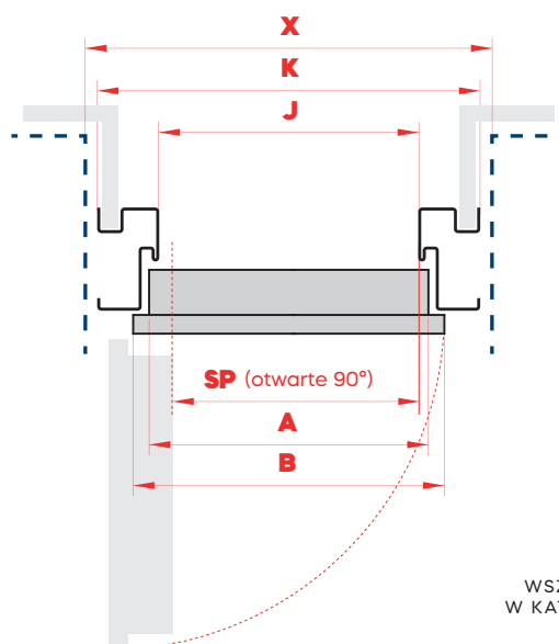
PRZEKRÓJ POZIOMY
