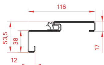
PROFIL OŚCIEŻNICY
